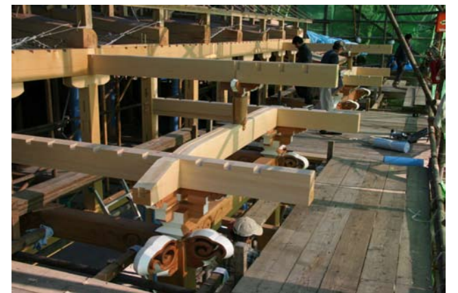
59 栴組の上に設置されたヒバ材の桁
