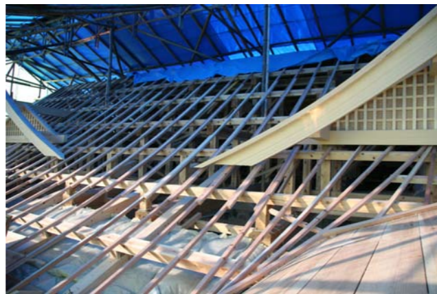
8 大屋根の反りに合わせて取り付けられた野垂木
