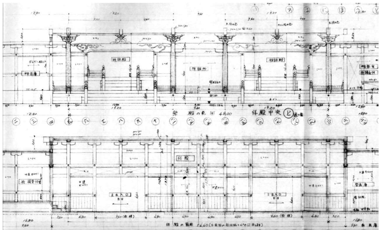
上段 社殿内部正面図 下段 社殿内部見返り図
