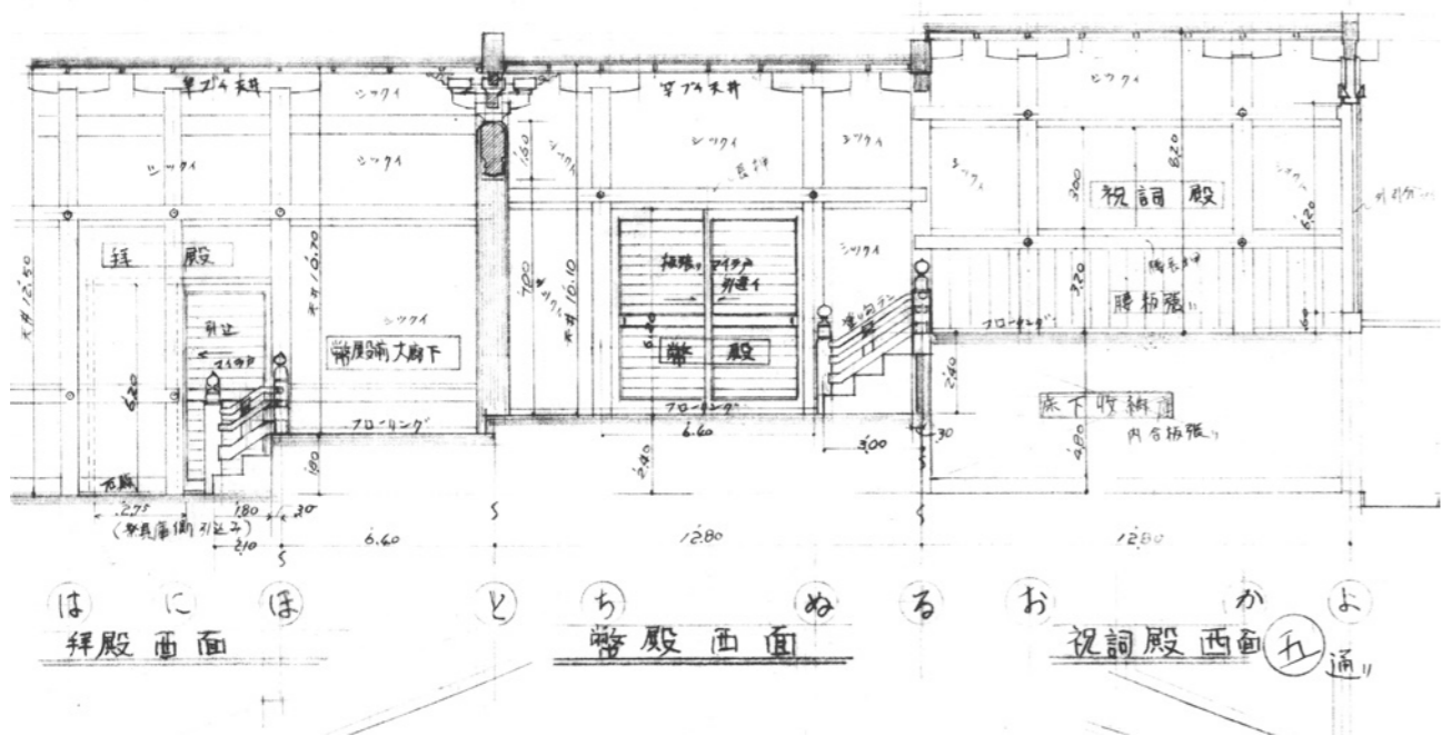
社殿内部側面図
